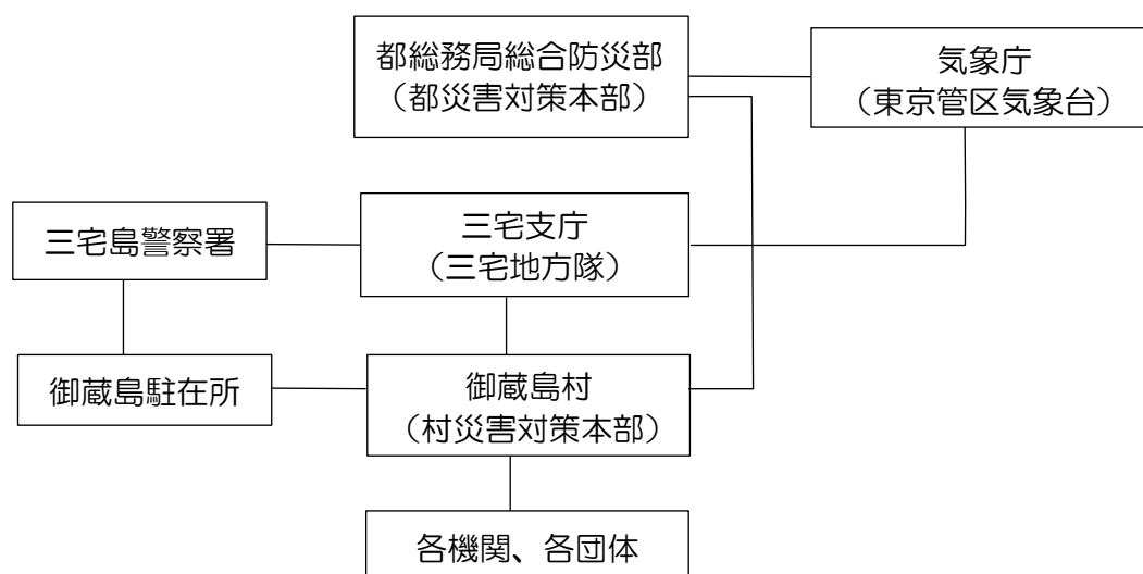
【通信系統図】
